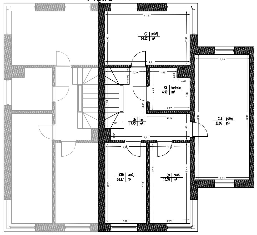
Piętro
