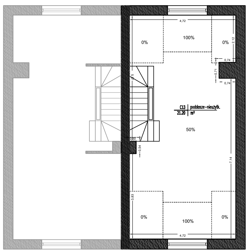
Poddasze nieużytkowe
